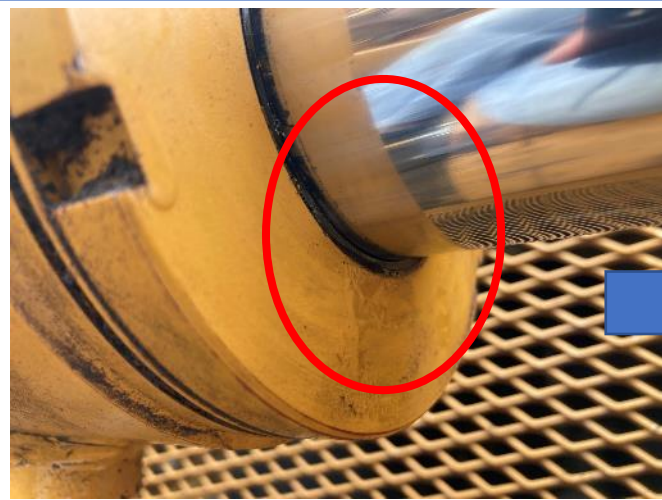
右ホッパーシリンダー油漏れ修理
