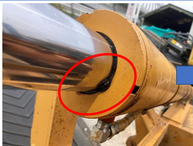
左ホッパーシリンダー油漏れ修理
