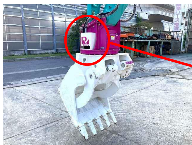
カバーに清掃窓の自作あり①
